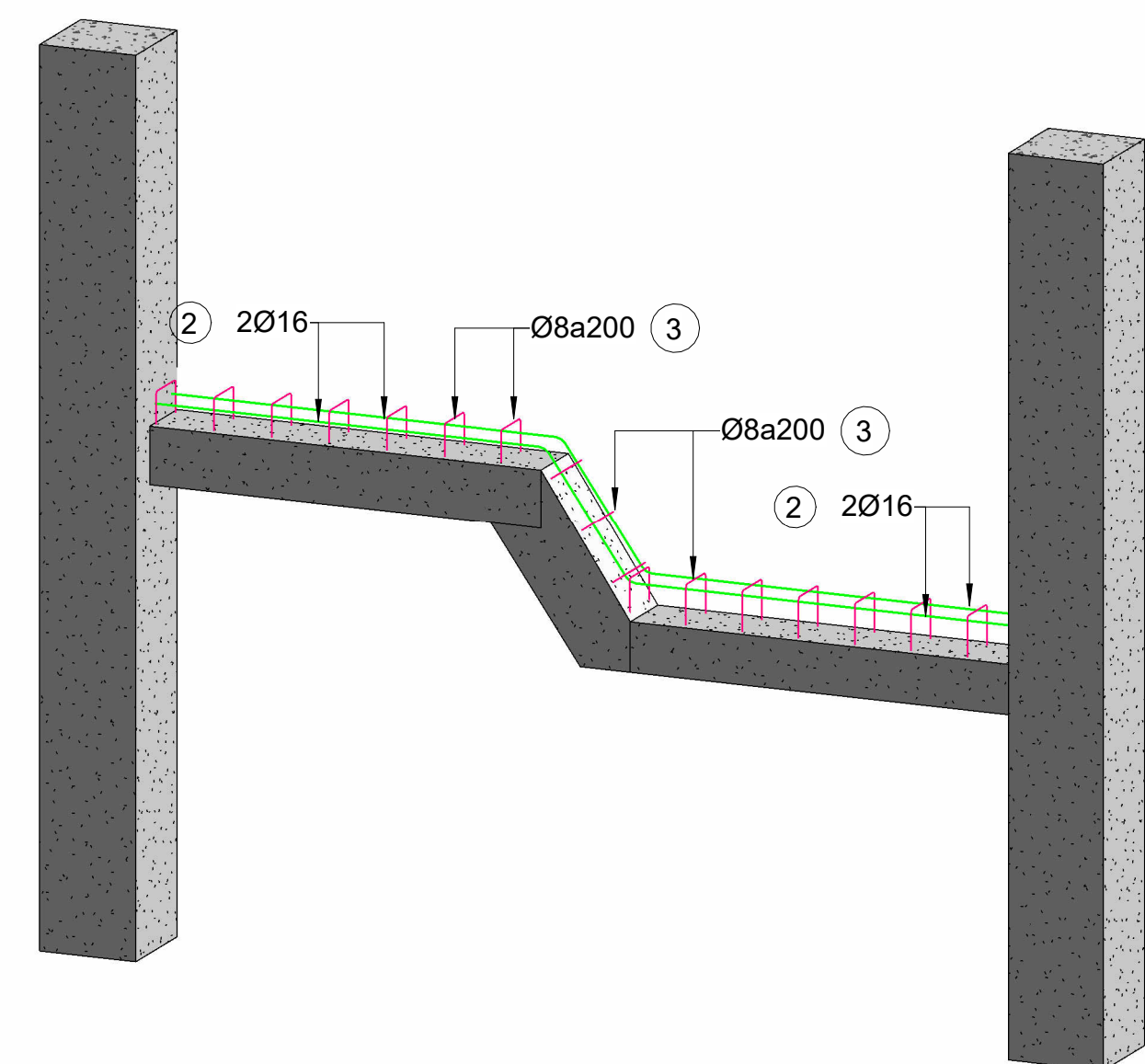
7 3D DẦM CHIỀU NGHỈ
