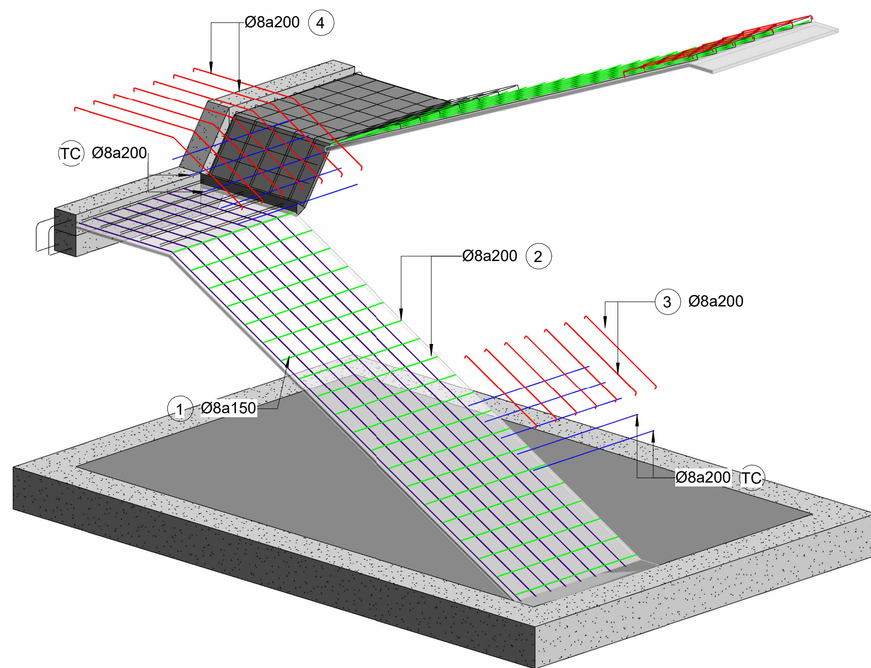
5 3D CẦU THANG BẢN 1
