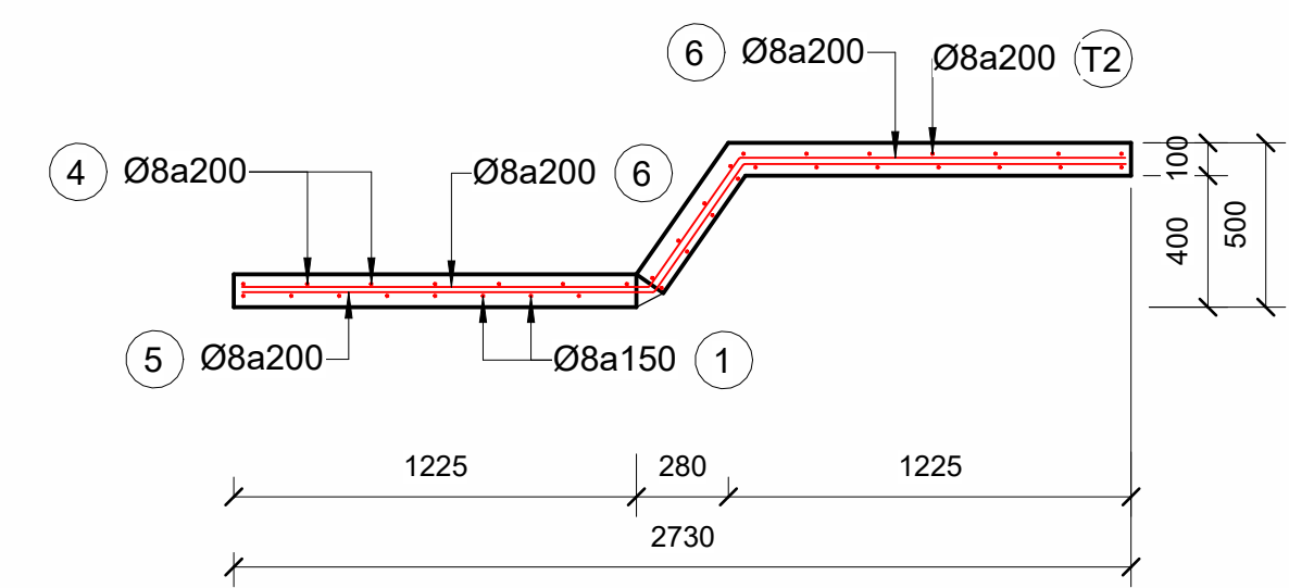
2 MẶT CẮT 2-2 1 : 25
