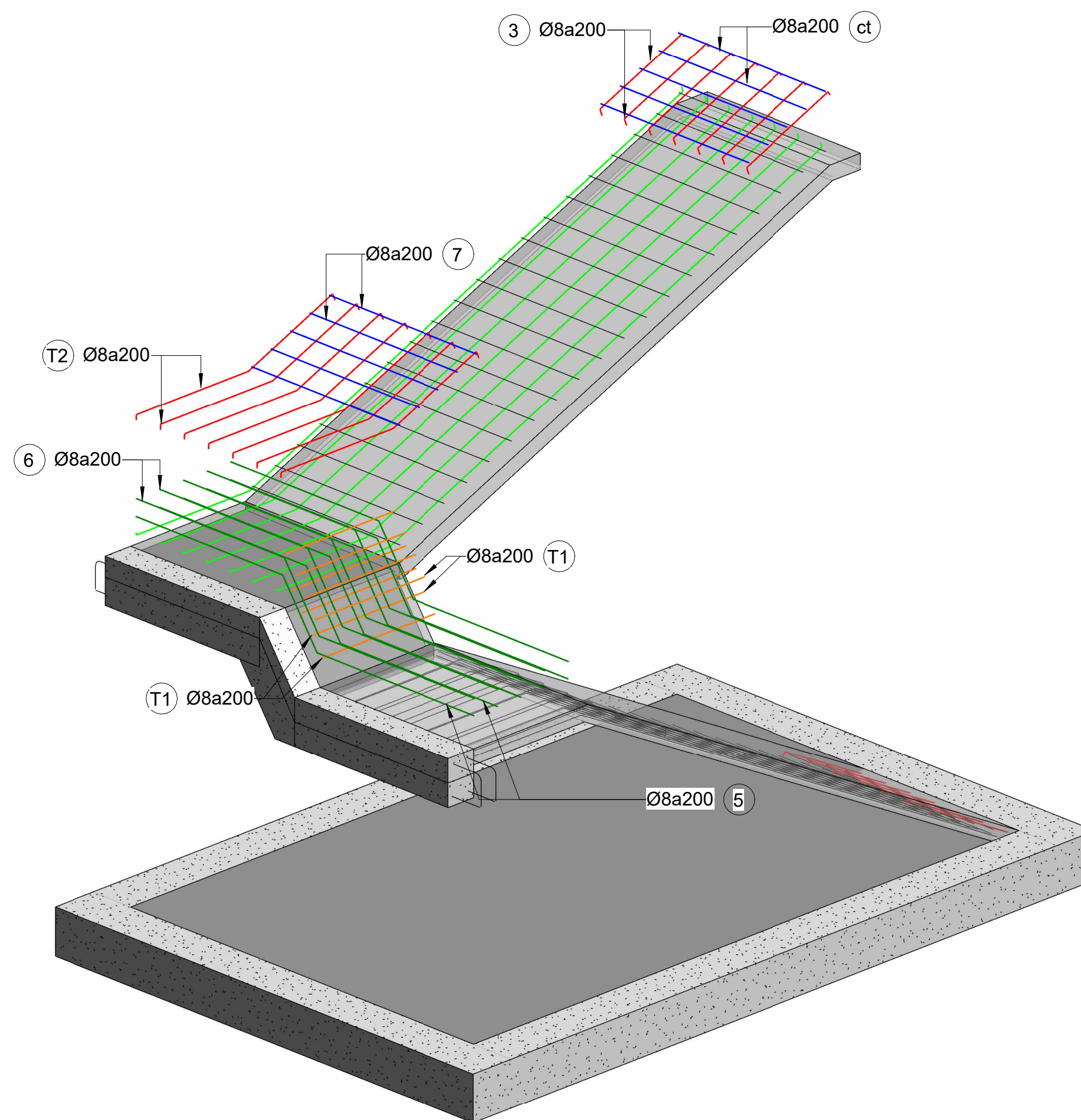
3 3D CẦU THANG BẢN 2
