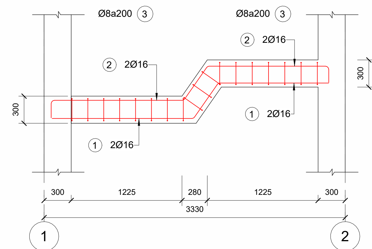
6 MẶT CẮT DẦM CHIỀU NGHỈ 1 : 25
