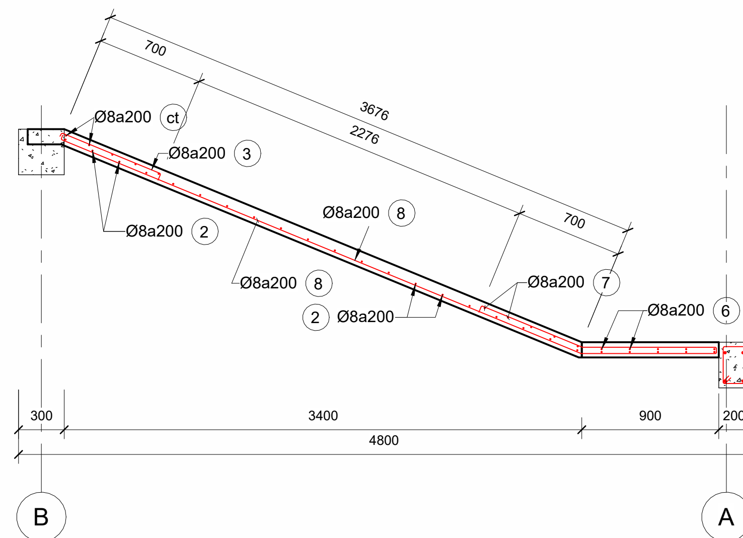
4 MẶT CẮT 3-3 1 : 25
